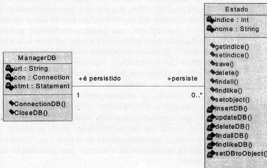
Figura 3 – Classe Estado com atributos e métodos do nível de aplicação e de persistência (primeiro modo)
