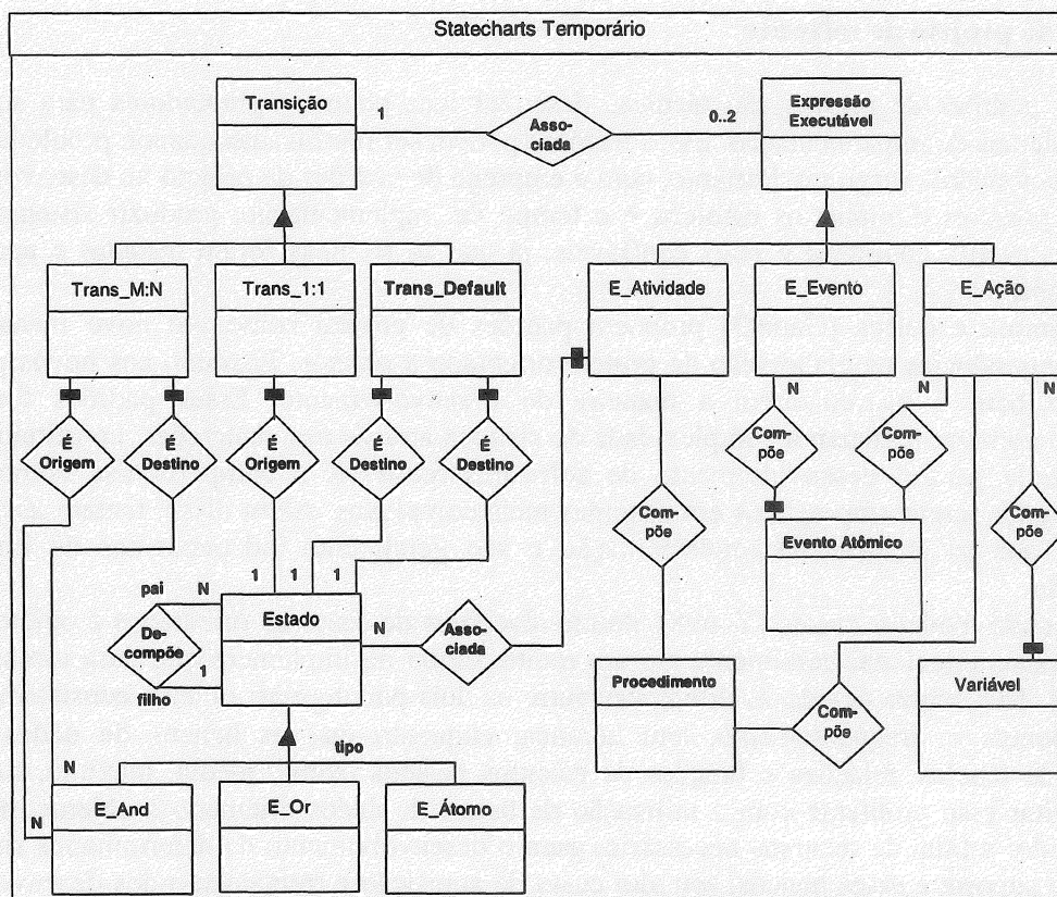
Figura 1 - Modelo de objetos do MAS para o tema statecharts temporário
